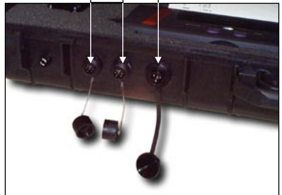
Detalle de Conectores exteriores para conexión de básculas, alimentación 12V y alimentación 220 V
